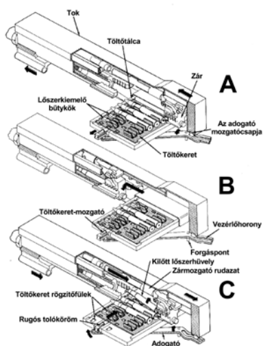
3. ábra: Vázlat az 5 cm Flak 41 adogatósi metódusáról
