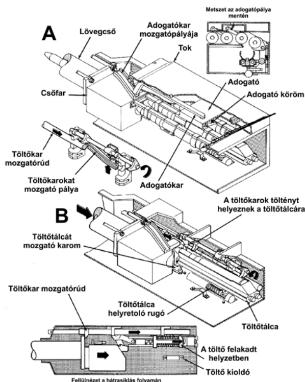
21. ábra: Az MK 412A géppágyú működési vázlat a az első két fázissal 34
