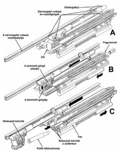
4. ábra: Vázlat az 5 cm Flak 41 ürítési metódusáról
