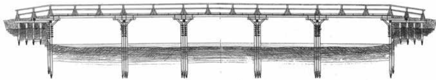
A 19. századi hidasnémeti fahíd hipotetikus szerkezeti vázlata (Molnár Ferenc rajza)
