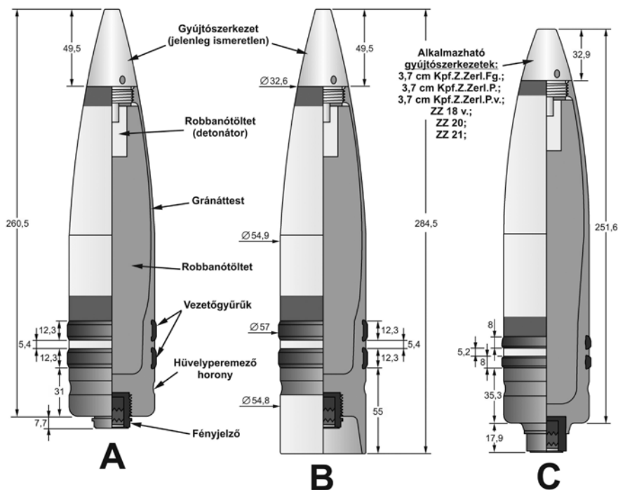
12. ábra: Rombológránátok (Minengeschoss) az 5,5 cm Gerät 58 légvédelmi gépágyúhoz
