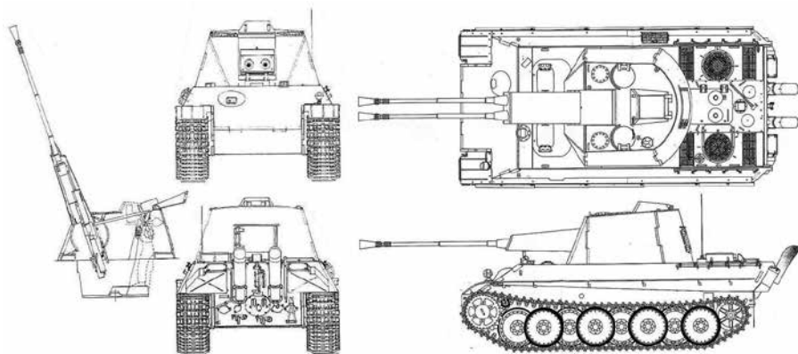
11. ábra: 5,5 cm Gerät 58 Zwillingflak Panther harckocsi alvázon. Egy a többféle Rheinmetall-terv közül 12
