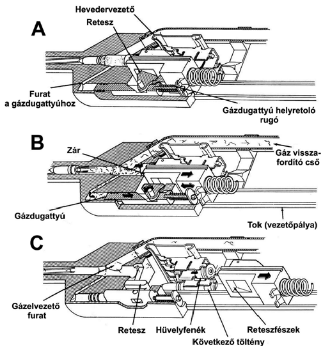
29. ábra: Az MK 115 gépágyú működési vázlat 49
