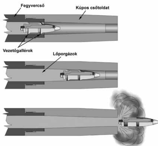
15. ábra: Elvi rajz az 5,5/4,1 cm tervezett kúpos csőtoldal működéséről Polte-féle galléros rombológránát esetén 18
