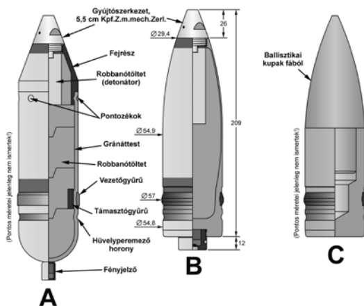
18. ábra: Rombológránátok 5,5 cm-es repülőgépfedélzeti fegyverekhez A - 1942-es korai, csak rajzon szereplő rombológránát; B - L/3,8 kaliberhosszú rombológránát; C - L/3,8 kaliberhosszú pótgránát 24
