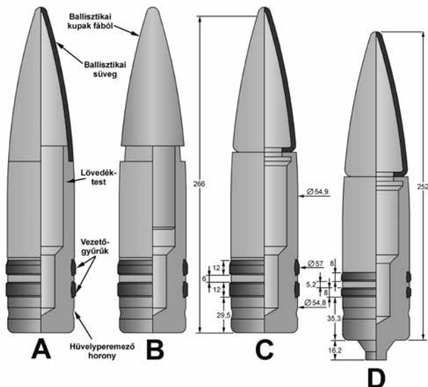
14. ábra: Pótgránátok az 5,5 cm Gerät 58 légvédelmi géppágyú kísérletekhez A - Pontozással rögzített lemezvas süvegű pótgránát (vezetőgyűrűk: 12 mm); B - Fakupakos pótgránát (vezetőgyűrűk: 12 mm); C - Dörzshegesztett lemezvas süvegű pótgránát (vezetőgyűrűk: 12 mm); D - Dörzshegesztett lemezvas süvegű pótgránát (vezetőgyűrűk: 8 mm) 15
