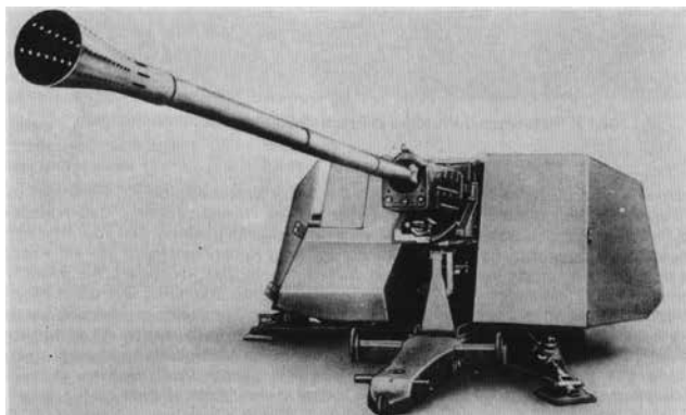
10. ábra: 5,5 cm Gerät 58 Rheinmetall-féle kísérleti géppágyú végleges változata tüzelőállásban 10
