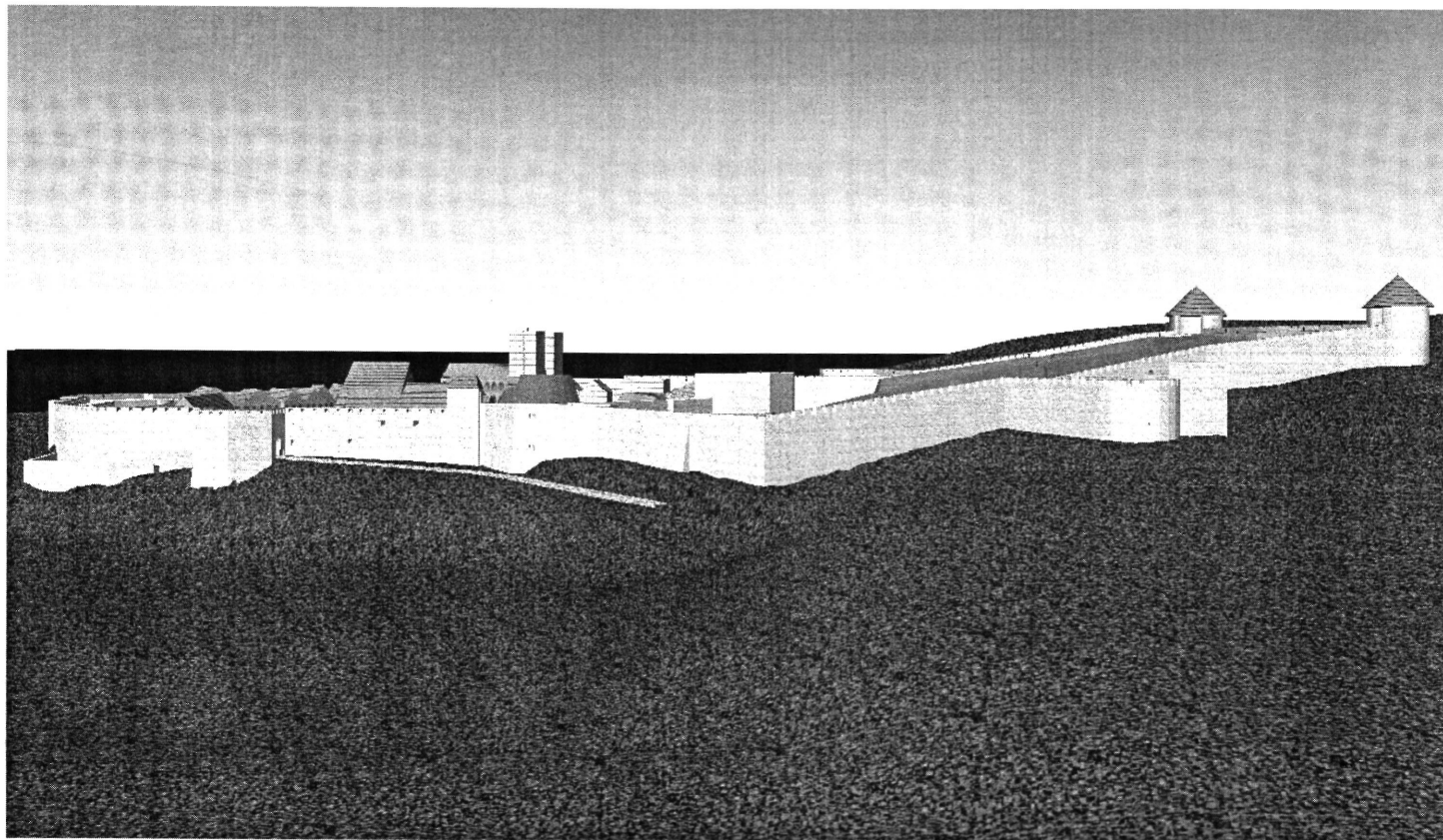
9. kép. Az egri vár számítógépes háromdimenziós modellje közelítőleg a Houfnagel-féle látkép nézőpontjából szemlélve. Mivel ez a modell az 1568-as állapotokat kísérli meg bemutatni, a Houfnagel-féle látkép elkészültéig a külső várban emelt védművek még nem láthatók.
