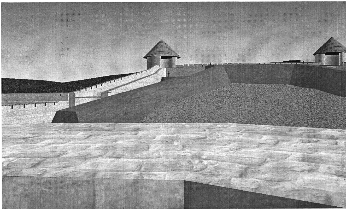
14. kép. Kilátás a külső vár és a környező dombok felé a Szentély-bástya tetejéről. Ez a minimális magasság, ahonnan még „közvetlen irányzással” tűz alá vehető az Almagyar-hegy tetején álló ostromló üteg.
